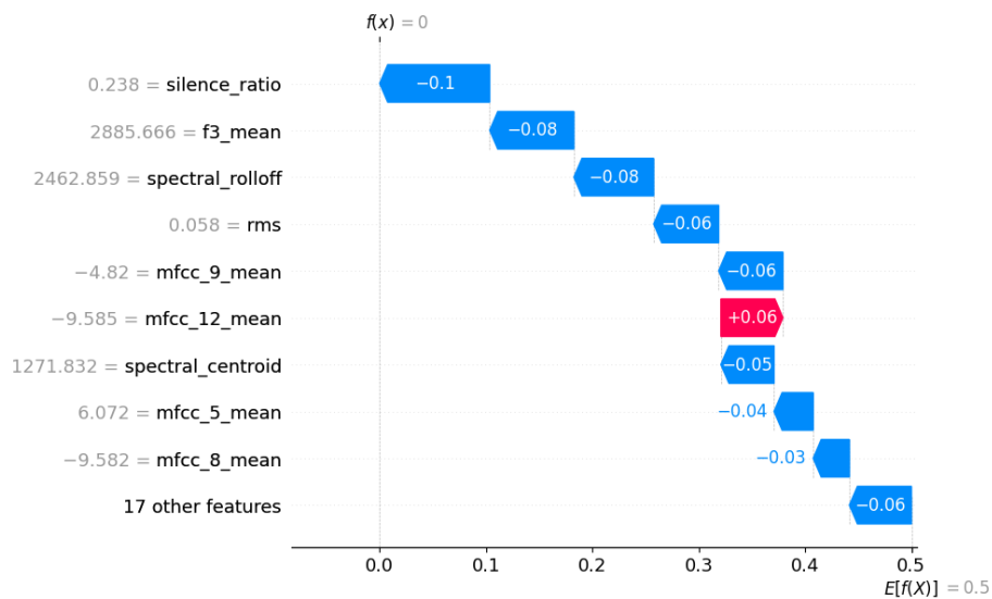
Figura 59: Explicación local con SHAP tras quitar spectral flatness, mfcc 1 y spectral bandwidth
